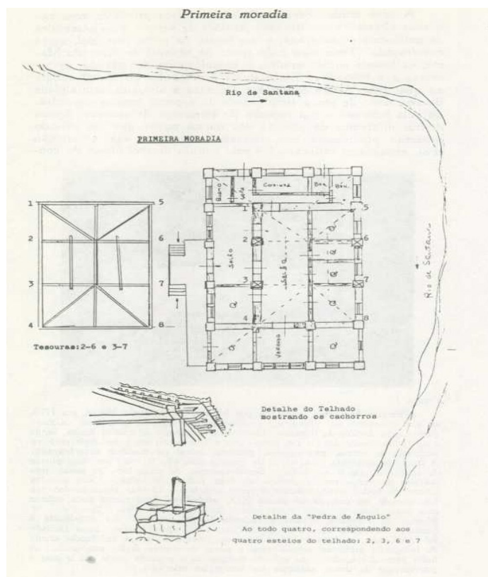
Figura 2. Planta da primeira casa da Fazenda Piedade
